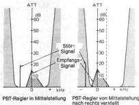
Abbildung 5-2: Verdeutlichung der Wirkungsweise der Bandbreitenregelung.
