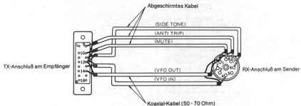
F) Abb. 5-5 Verbindungskabel für Sender und Empfänger (HF)
